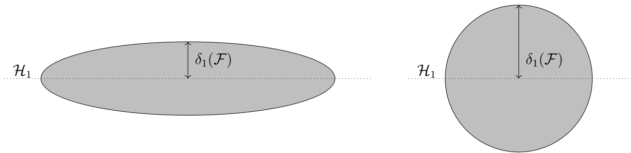
FIGURE 2.1 – Largeur de Kolmogorov d'ellipses en dimension 2. Une ellipse allongée est mieux approchée par un sous-espace linéaire de dimension 1 qu'un boule (la pire des familles). La largeur de Kolmogorov capture donc la courbure de familles de fonctions.
