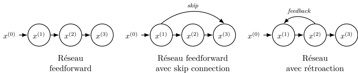
FIGURE 1.4 – Exemples d’architectures communes de réseaux de neurones. Chaque flèche horizontale indique une application \mathcal{A}_j . Les flèches feedback et skip indiquent que l’information d’une couche est transportée à une autre couche.
